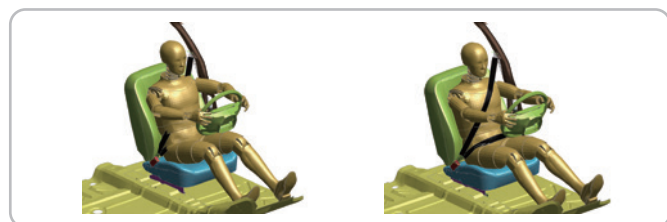
ダミーポジショニング/シートベルトフィッティング
