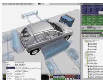
複数モデルセットアップ機能
